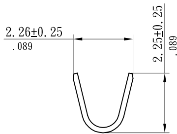
A-A SECTION
