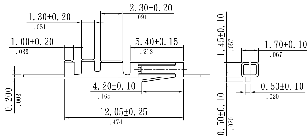
SECTION D-D
